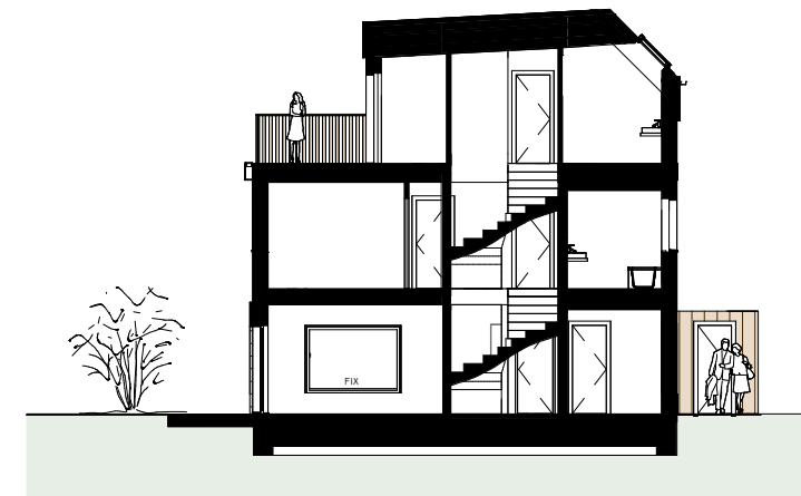
LÄNGSSCHNITT
