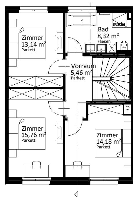
1. Obergeschoß
