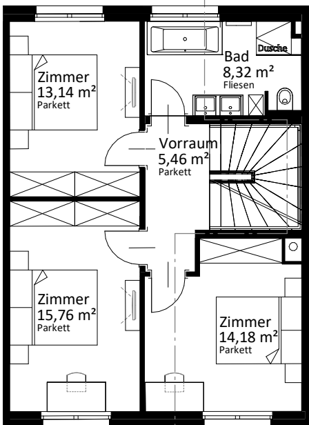
1. Obergeschoß
