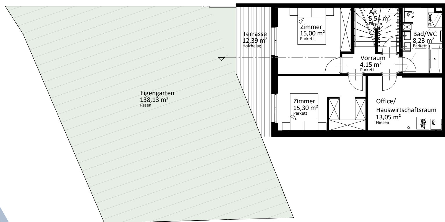
Untergeschoß
