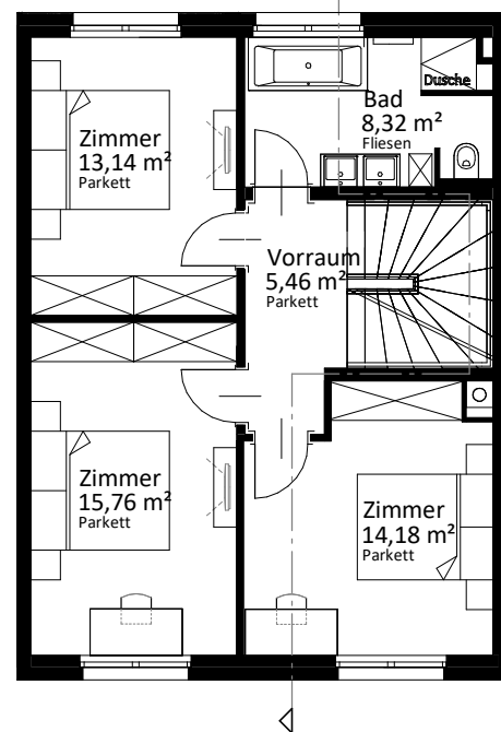
1. Obergeschoß
