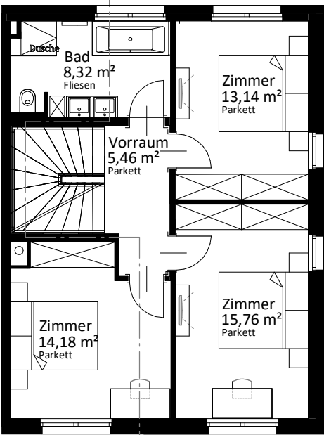
1. Obergeschoß
