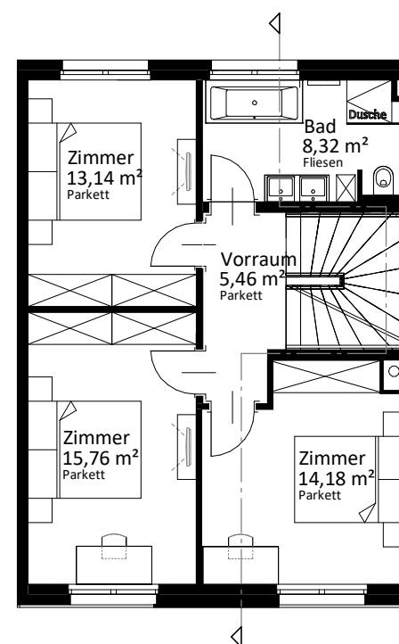
1. Obergeschoß
