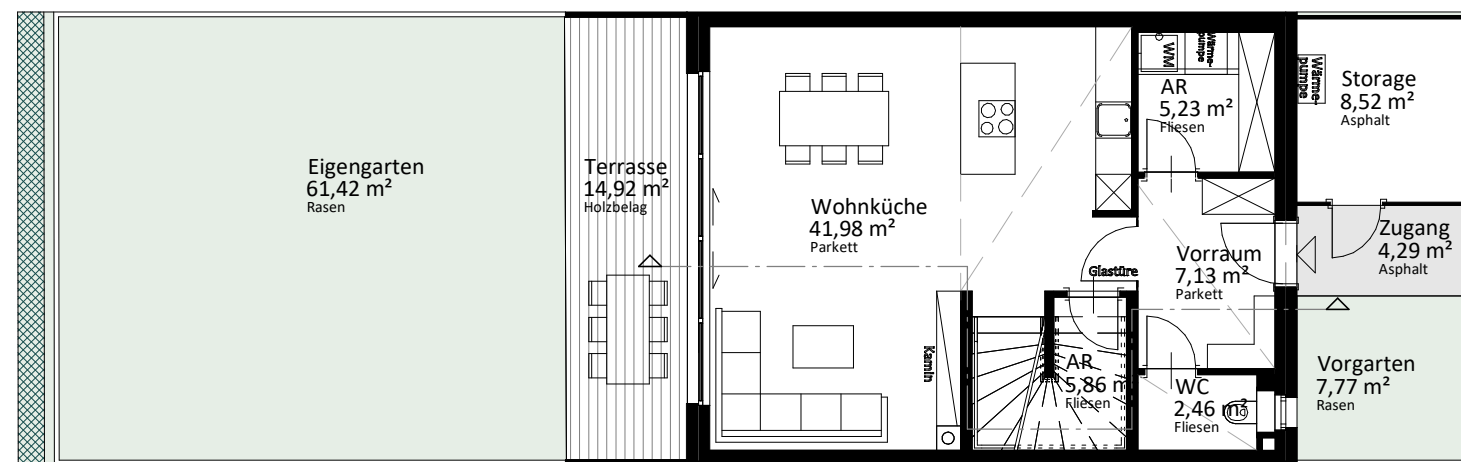
Erdgeschoß
