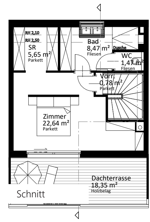
2. Obergeschoß
