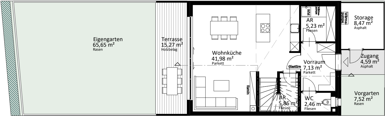
Erdgeschoß
