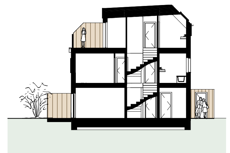
Schnitt
