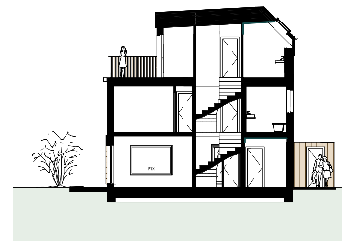
Schnitt
