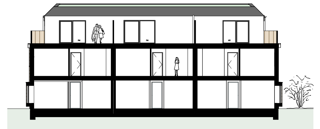
LÄNGSSCHNITT
