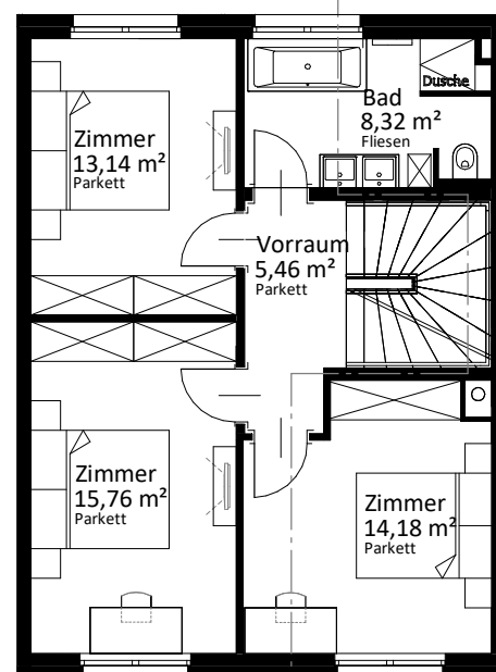
1. Obergeschoß
