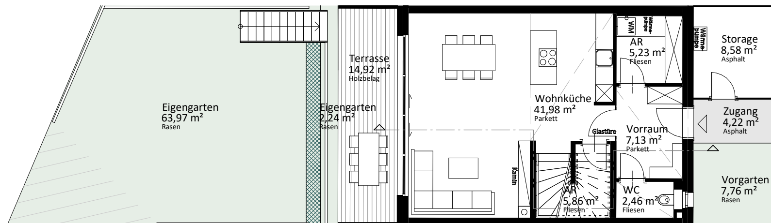
Erdgeschoß
