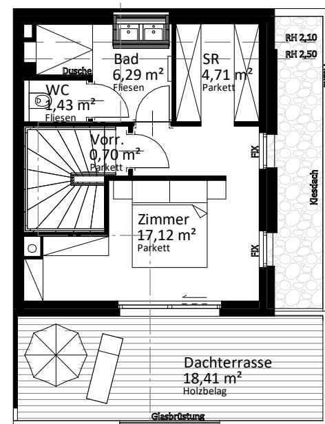
2. OBERGESCHOß 2. Obergeschoß
