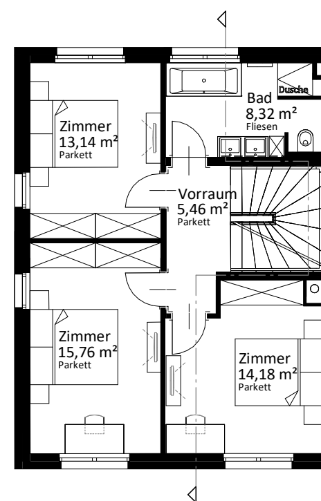
1. Obergeschoß
