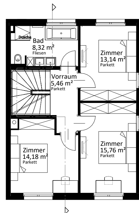
1. Obergeschoß
