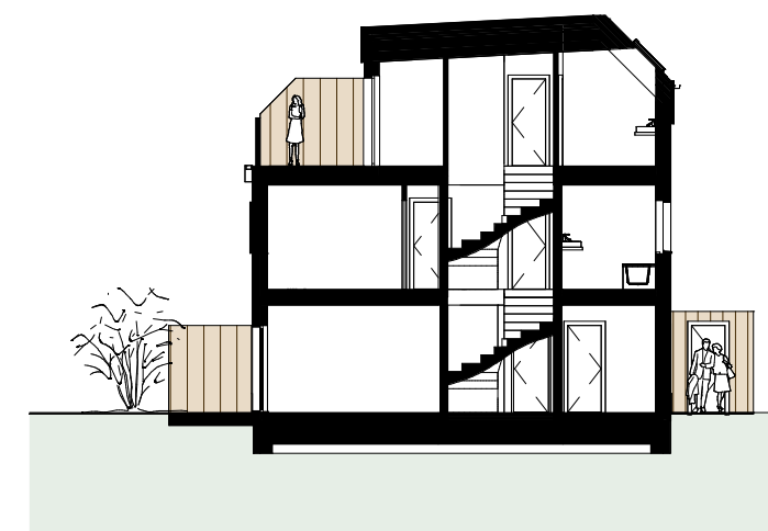
Schnitt
