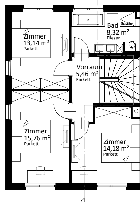
1. Obergeschoß
