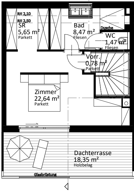
2. Obergeschoß
