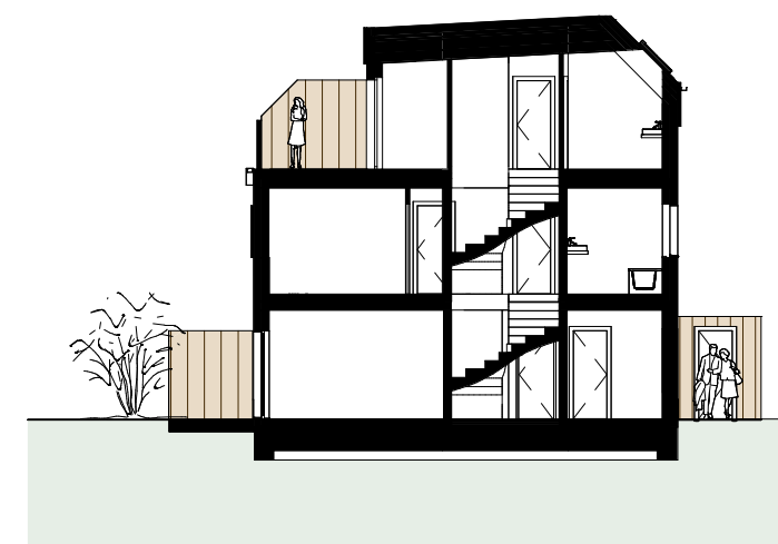
Schnitt
