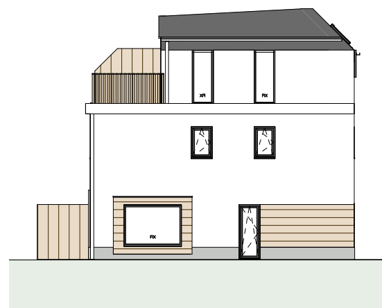
ANSICHT - H3
