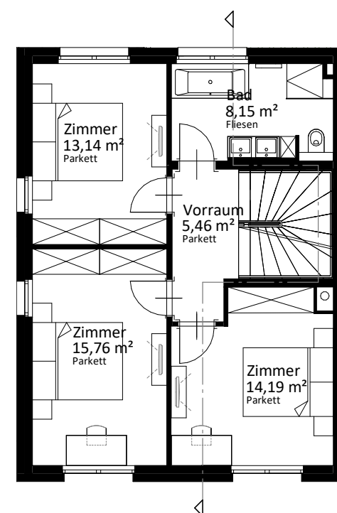
1. Obergeschoß
