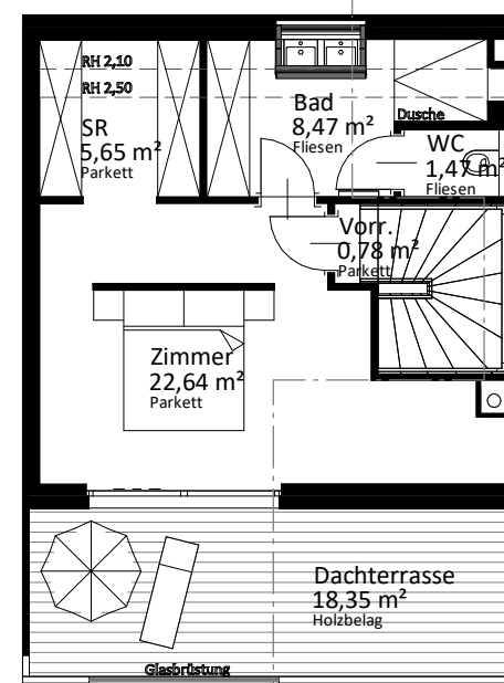
2. Obergeschoß
