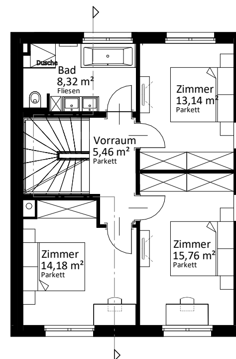
1. Obergeschoß
