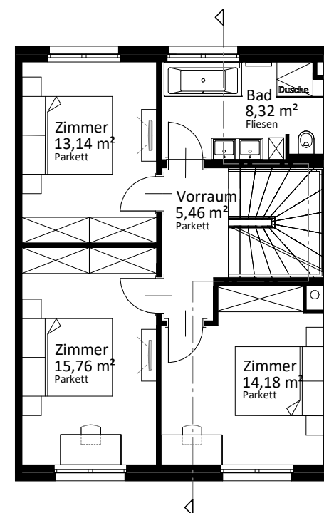
1. Obergeschoß
