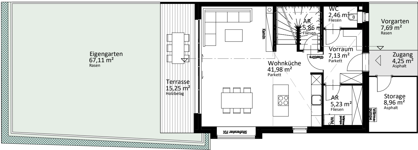
Erdgeschoß
