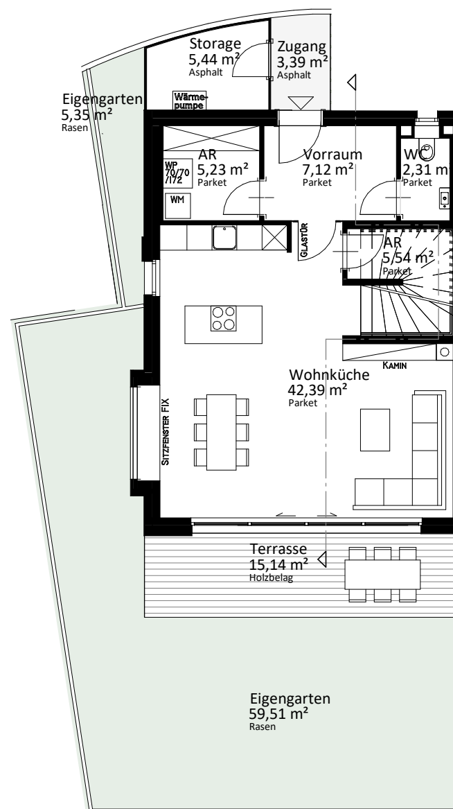
Erdgeschoß
