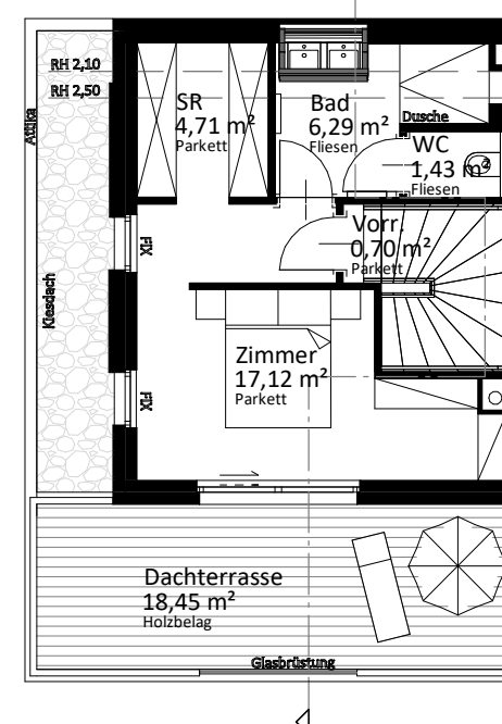
2. Obergeschoß
