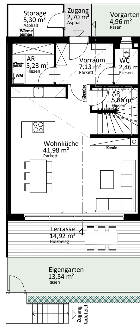
Erdgeschoß
