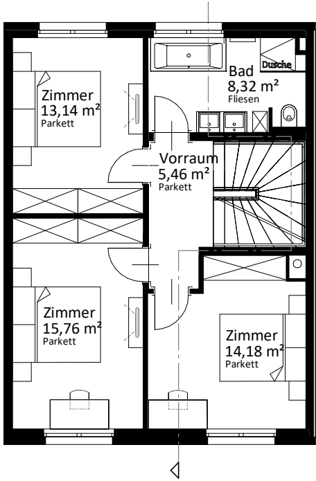
1. Obergeschoß
