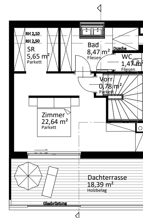
2. Obergeschoß
