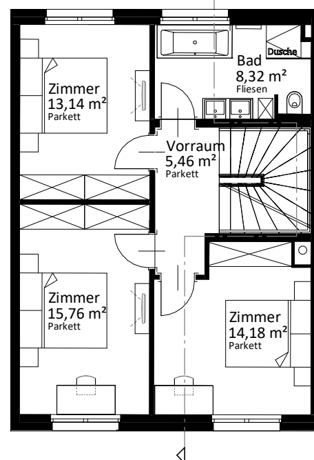
1. Obergeschoß
